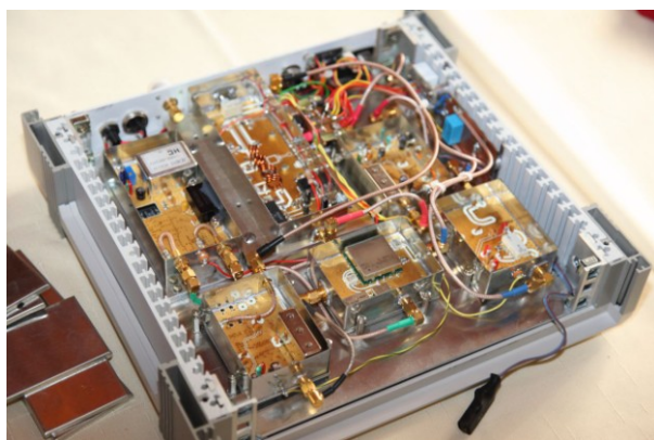
144-MHz-Transverter
