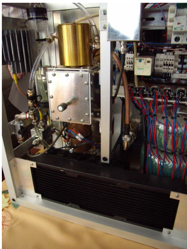
0,8 kW-PA für 23 cm von OL3Z
